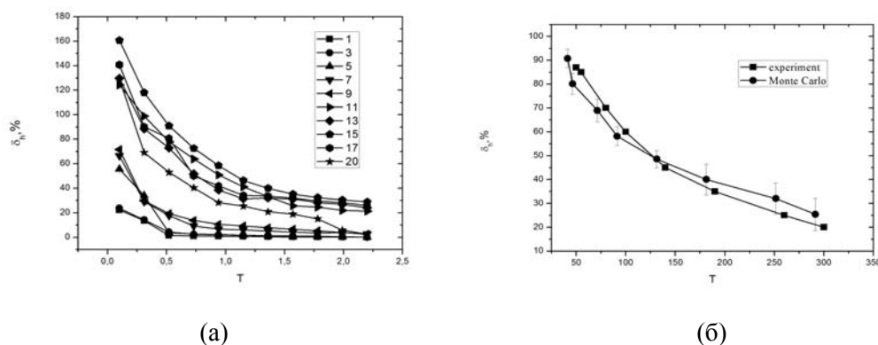
Рис 1. Зависимость коэффициента магнитосопротивления трехслойной структуры, состоящей из двух ферромагнитных слоев, разделенных немагнитным слоем, от температуры для различных значений толщины N ферромагнитных пленок (а), и сопоставление графиков температурной зависимости коэффициента магнитосопротивления для структуры Fe/Cr при толщине пленок железа в 3 нм (б), рассчитанных методами Монте-Карло и измеренных экспериментально [1].
