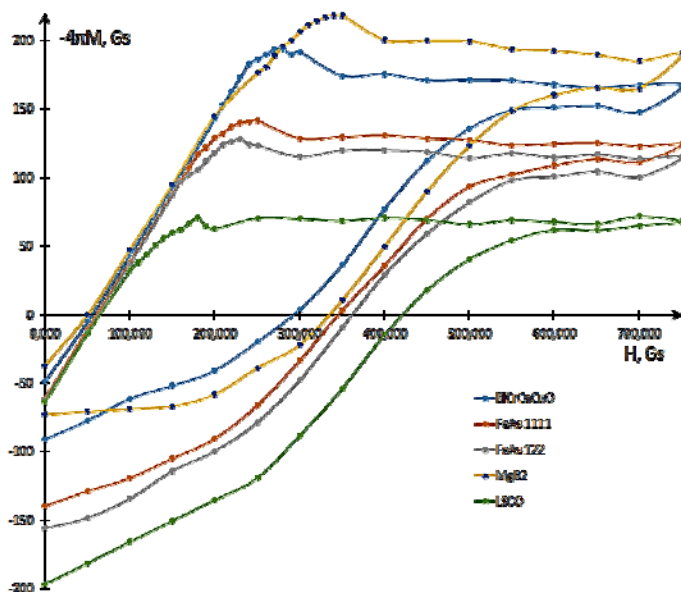
Рис 1. Намагниченности сверхпроводящих образцов с 700 дефектами
