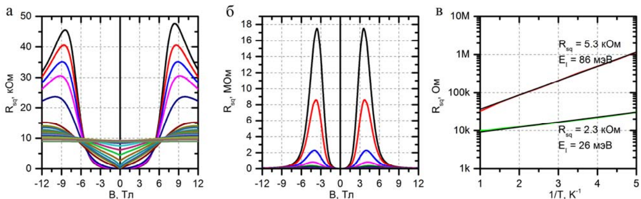
Рис. 1. Магнитопольевые зависимости сопротивления двух пленок с (а) R_{sq} = 2.3 кОм и (б) R_{sq} = 5.3 кОм при температурах от 0.2 К до 6.6 К; (в) Зависимость сопротивления в активационных координатах в магнитном поле B = 6.9 Тл.
